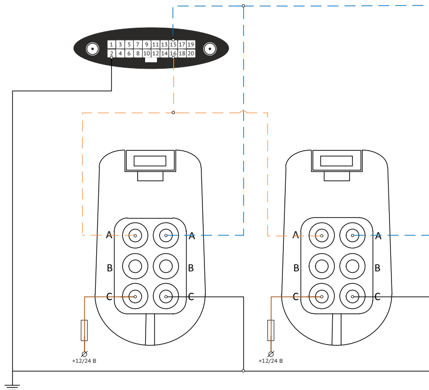
Рисунок 63. Схема подключения двух топливных датчиков Omnicomm LLS-AF20160
