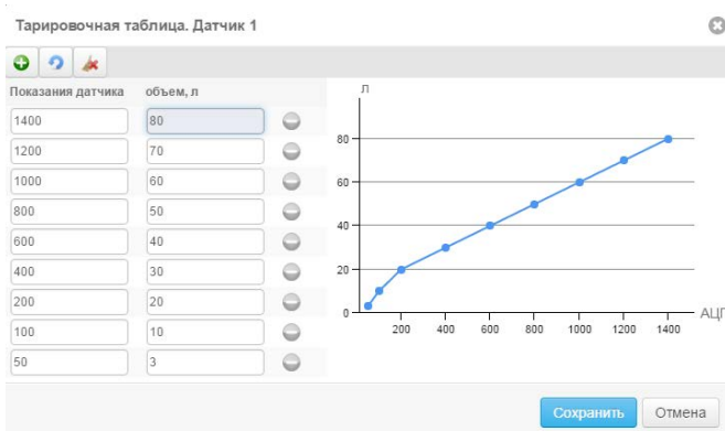
Рисунок 64. Тарировочная таблица
