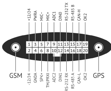
Рисунок 57. 20-контактный разъем трекера
