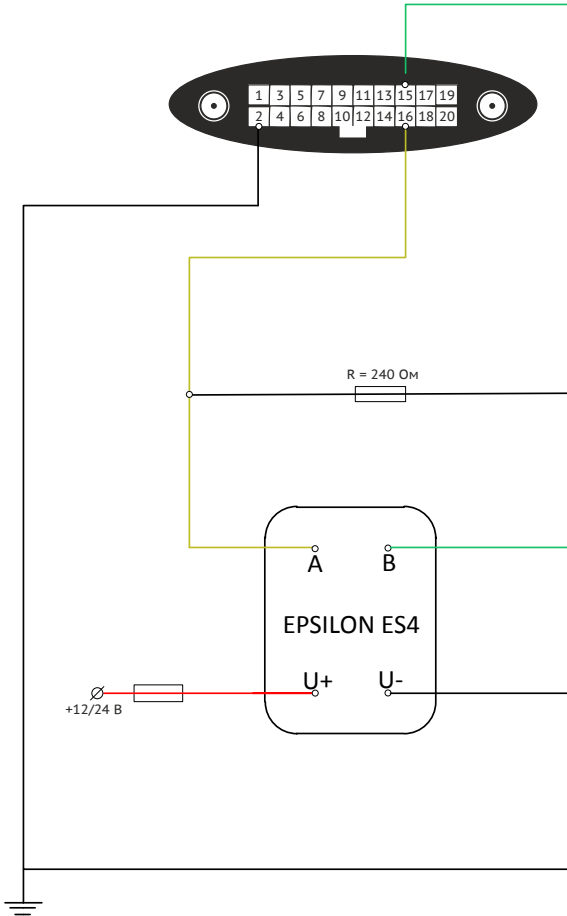
Рисунок 66. Схема подключения топливного датчика ES4
