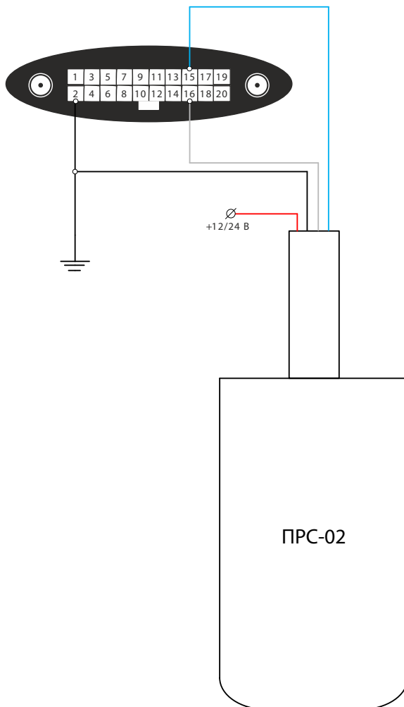
Рисунок 60. Схема подключения датчика контроля работы экскаватора
