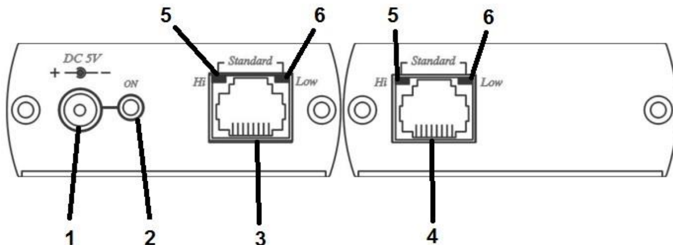
Рис. 2 Вид спереди
