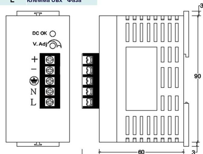
Габаритные размеры AD1048FS и обозначения на передней панели
