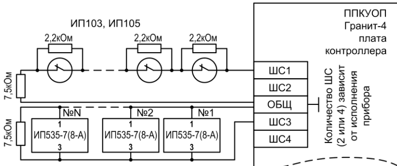
Рис.Б4 Схема подключения ручных пожарных извещателей ИП535-7, ИП535-8-А и тепловых пожарных извещателей типа ИП103, ИП105
