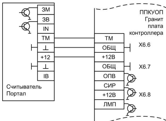
Рис.Б7 Схема подключения считывателя «Портал»
