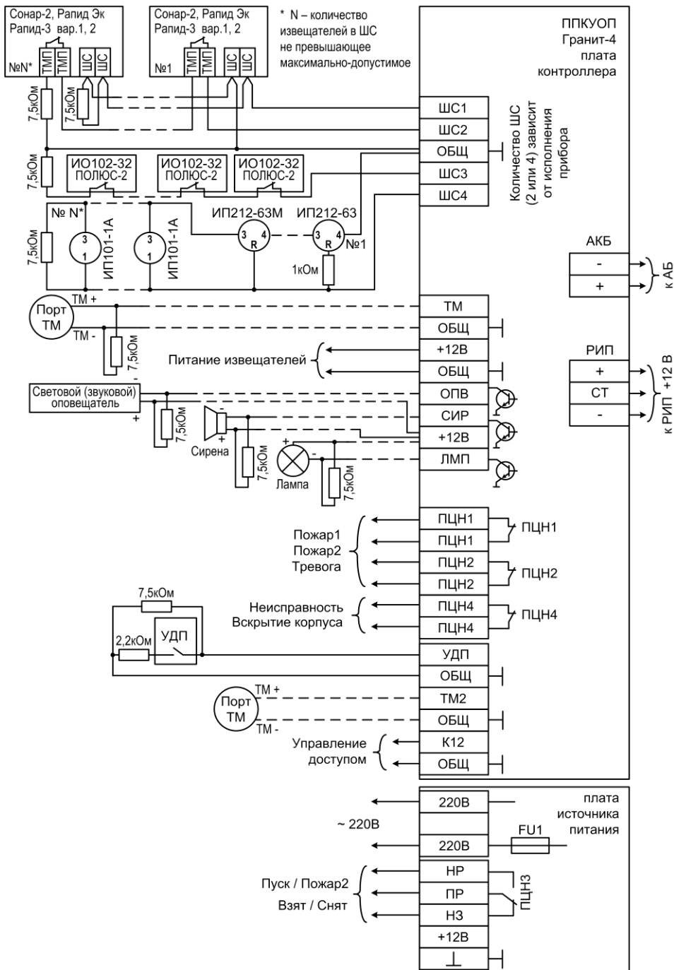
Рис.Б2 Схема внешних подключений
