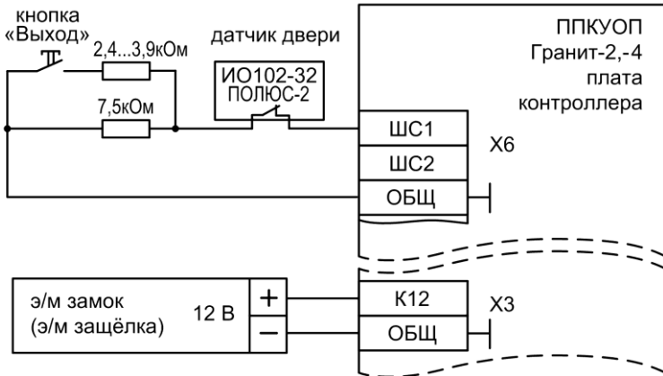
Рис.Б3 Схема подключения цепей управления доступом и э/м замка (э/м защёлки)
