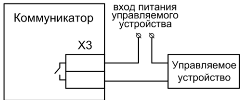
Рис.4 Схема подключения внешнего управляемого устройства к коммуникатору
