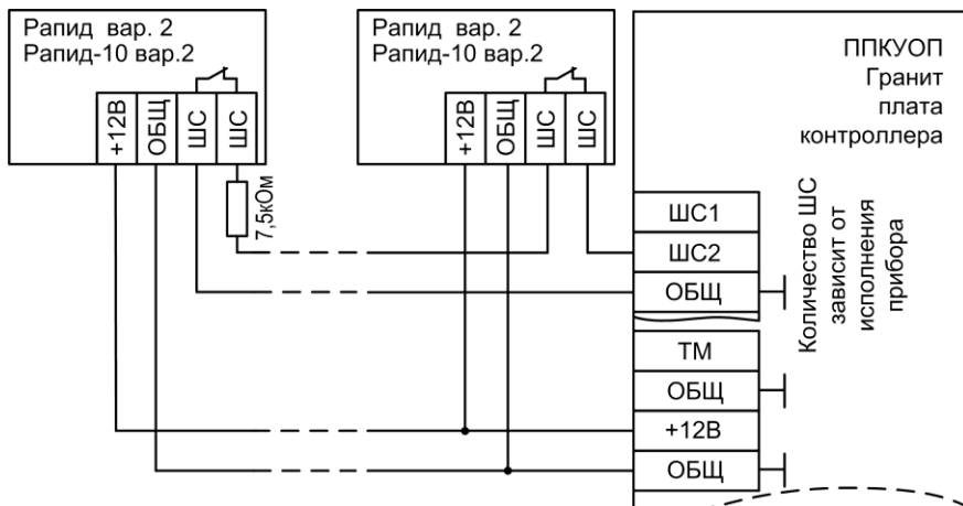
Рис.Б6 Схема подключения охранных извещателей Rapid вар.2, Rapid-10 вар.2
