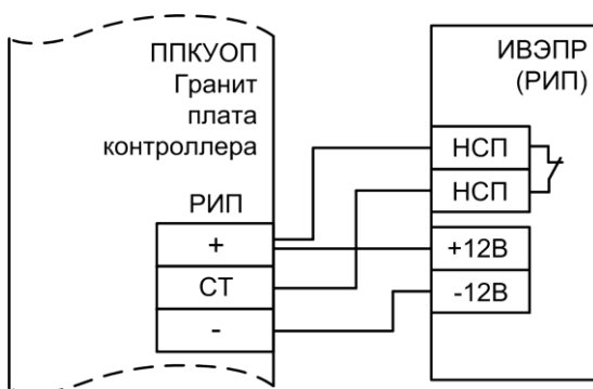
Рис.Б8 Схема подключения источника внешнего электропитания резервированного (РИП)
