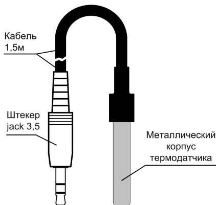
Рис.6 Термодатчик «DS18B20 L=1,5м, jack 3,5 мм». Общий вид
