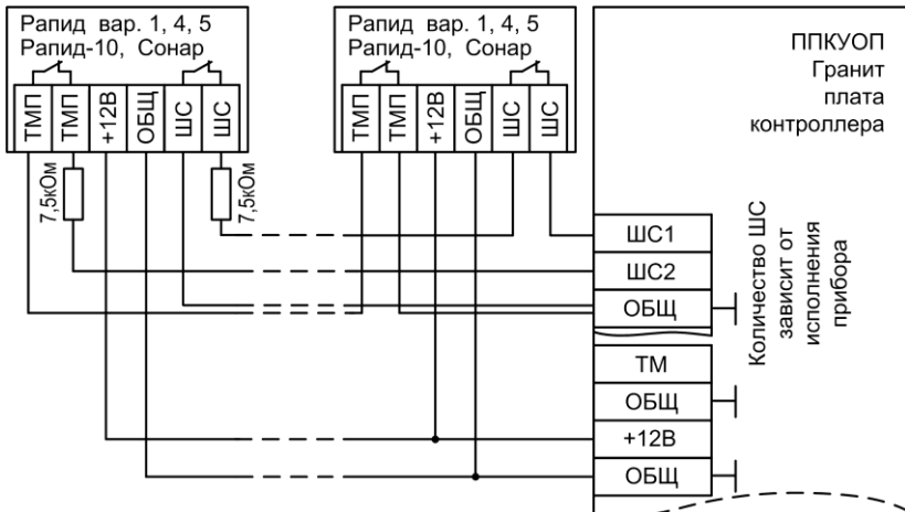
Рис.Б5 Схема подключения охранных извещателей Rapid вар.1,4,5, Rapid-10, Сонар (тампер подключён к отдельному ШС)
